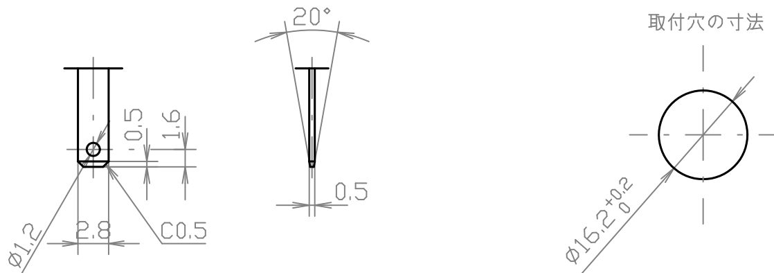
寸法詳細2/1
