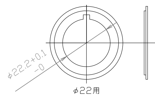
C3604 t=1.6 Niメッキ仕上げ
