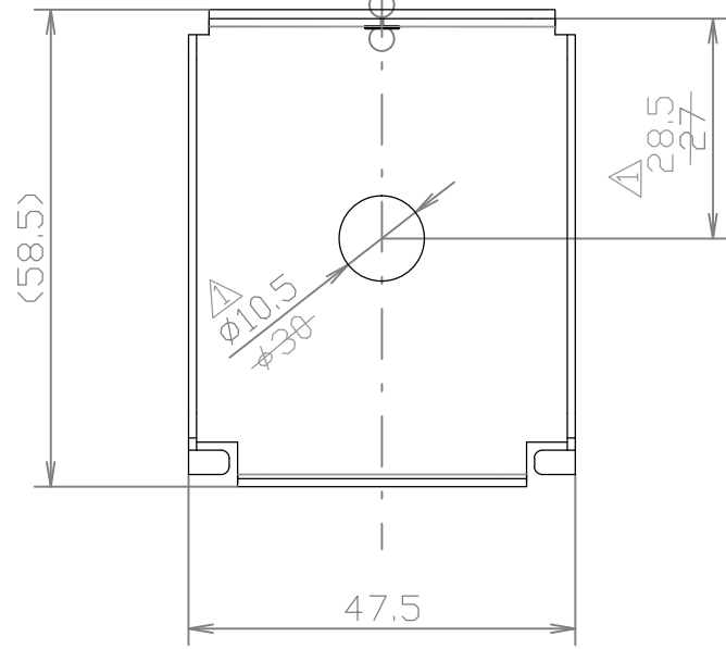
付属アダプターリング
